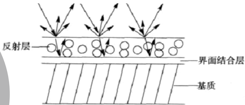
图1 太阳热反射隔热涂层作用示意
