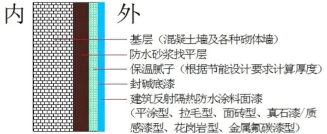
有墙面保温腻子的建筑反射隔热防水涂料系统外墙施工基本构造
